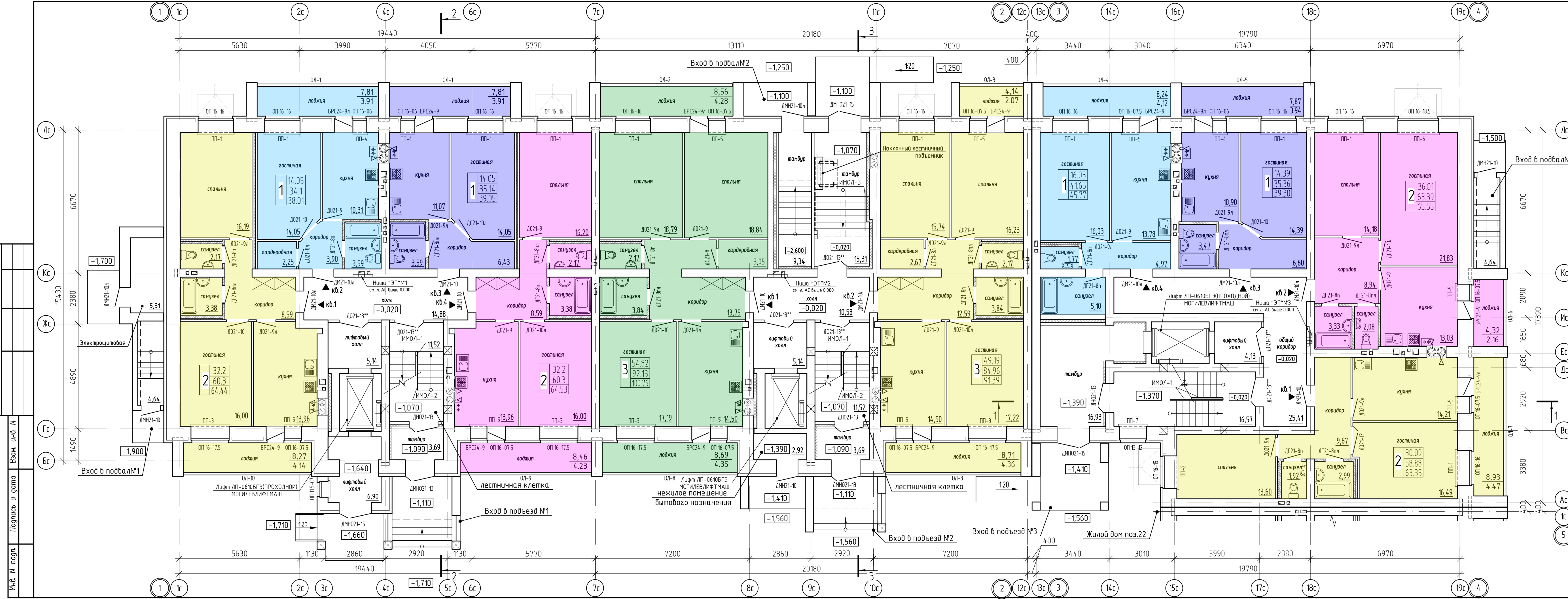
Показатели на 1-ый этаж в осях 1с-7с
